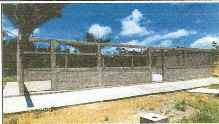
FOTO 2: Se observa la necesidad de instalar ventanas tipo balcon para poder brindar seguridad y ventilacion al aula
